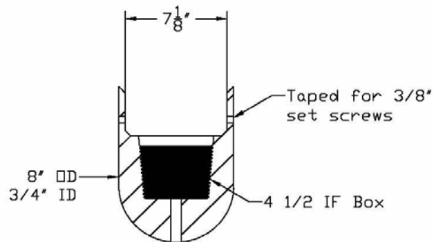
UHMW Bottom Section
