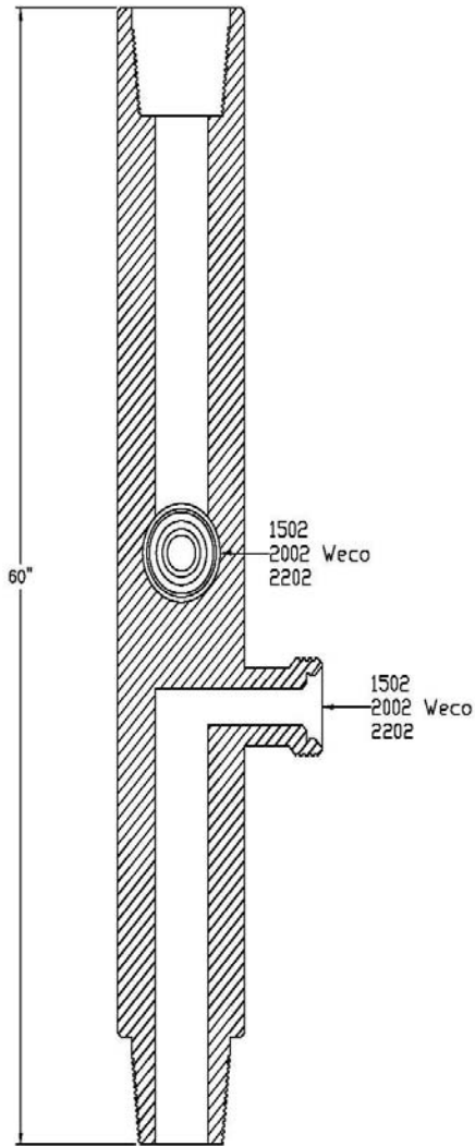
Double Weco Top Test Mandrel (DWTTs)
