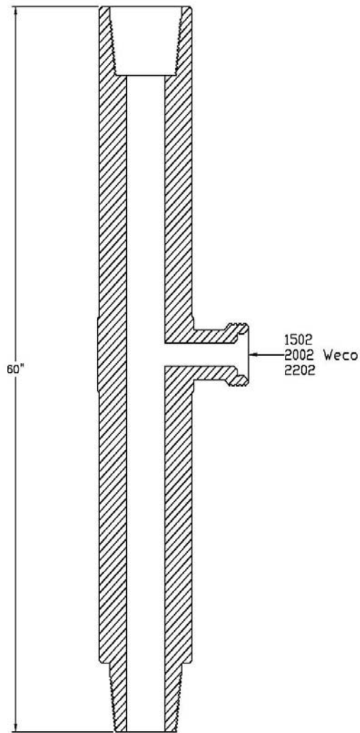
Top Test Mandrel (TTS)
